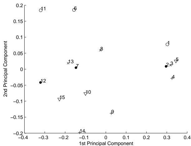
Fig. 9. PCA
