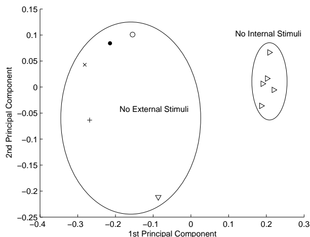
Fig. 8. PCA
