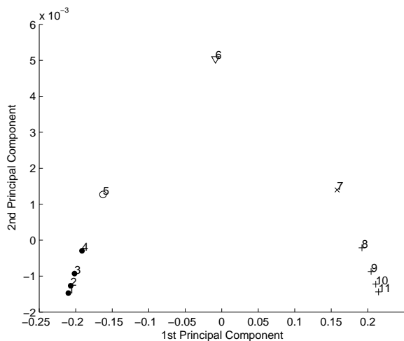
Fig. 7. PCA
