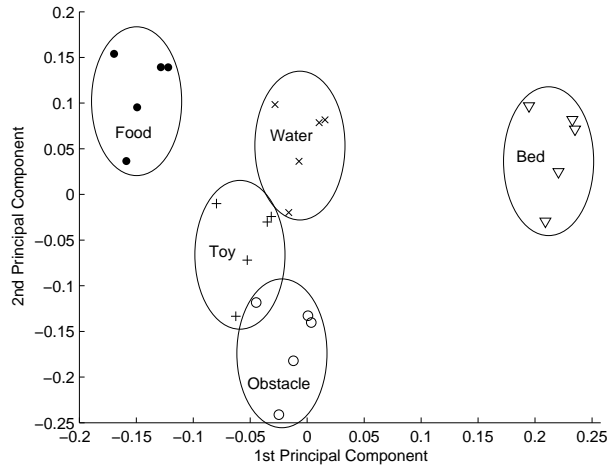
Fig. 6. PCA
